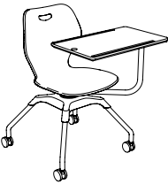
No Rack W28½" D28-34" H33⅜" Seat: W17⅜" D20" H18½"
